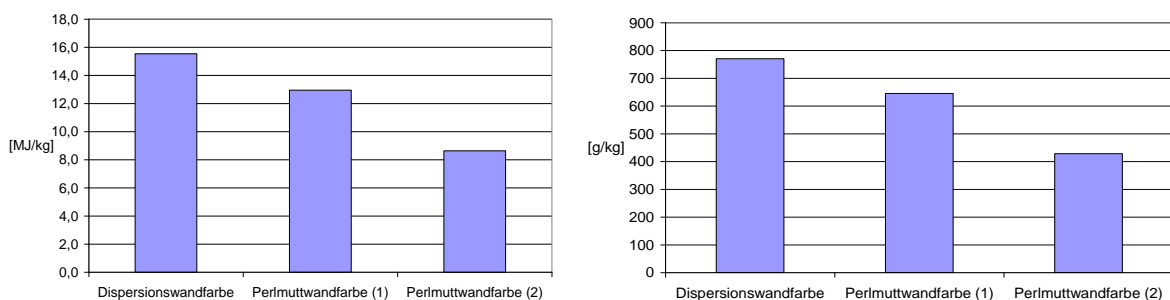
Abb. 3 Primärenergieäquivalente [MJ] und CO 2 -Emissionen [g] für die Herstellung von 1 kg Wandfarbe (inkl. CO 2 aus nicht erneuerbaren Rohstoffen) 1
