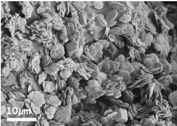
Abb. 2 Rasterelektronenmikroskopisches Bild von Calciumcarbonatkristallen, die mit Hilfe einer neuen Apparatur in eine Matrix aus Chitin kristallisiert wurden.
